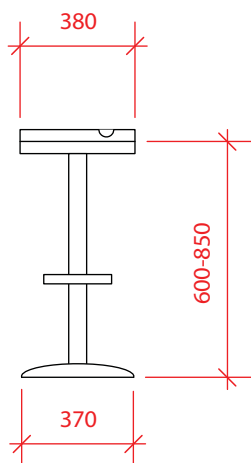
Ansicht Vorne
